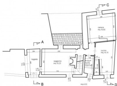
PIANTA PIANO TERRENO
