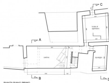
PIANTA PIANO PRIMO SOTTOSTRADA
